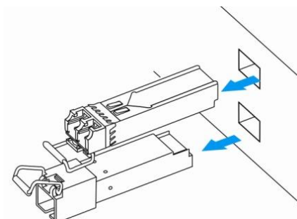
Рисунок 41 – Извлечение SFP-трансиверов
