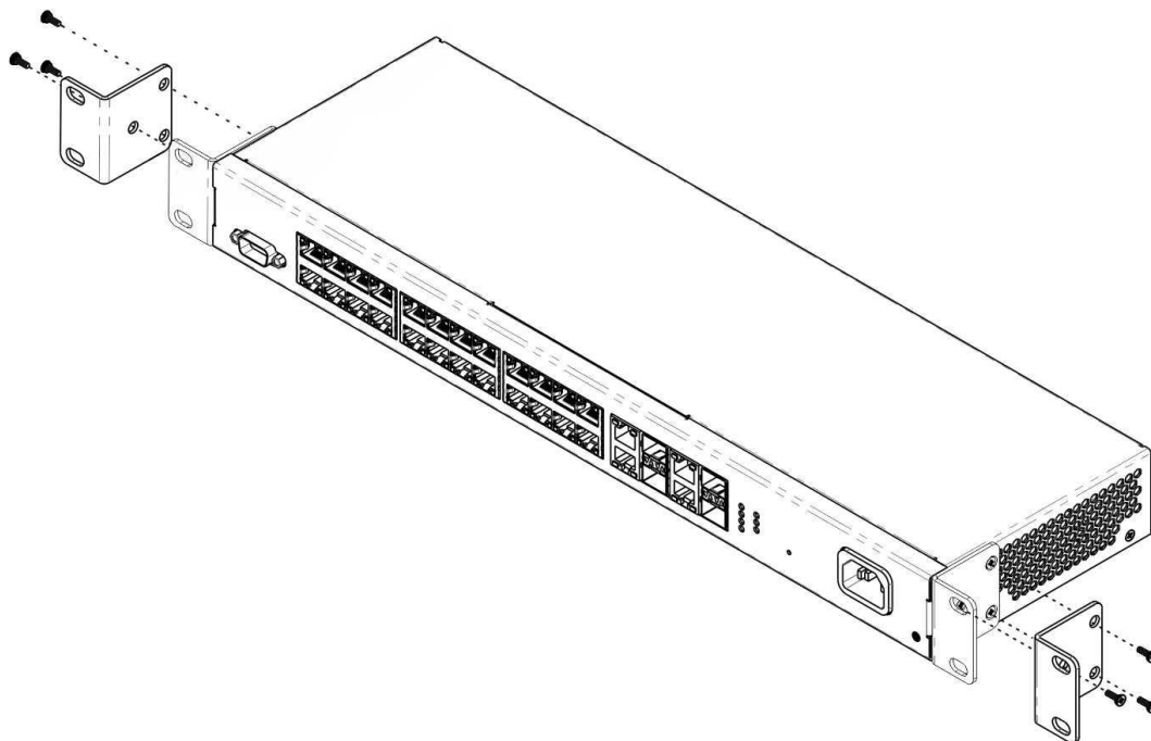
Рисунок 35 – Крепление кронштейнов
