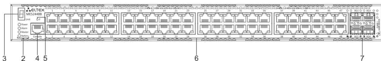
Рисунок 20 – Передняя панель MES2448B
