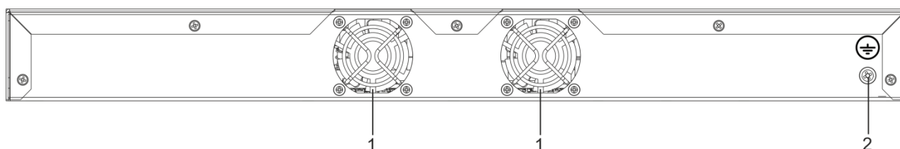
Рисунок 25 – Задняя панель коммутатора MES2428P
