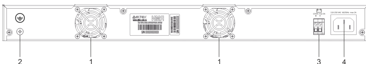
Рисунок 27 – Задняя панель коммутатора MES2448B
