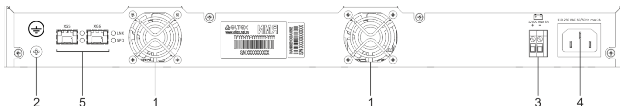
Рисунок 28 – Задняя панель коммутатора MES2448E
