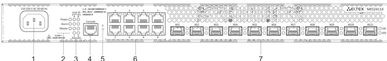
Рисунок 22 – Передняя панель MES2411X
