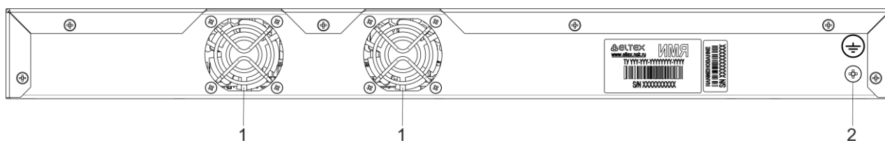
Рисунок 29 – Задняя панель коммутатора MES2411X
