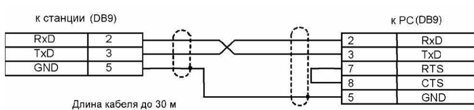
Рисунок 27 – Схема кабеля для подключения к ПОРТ1, ПОРТ2
