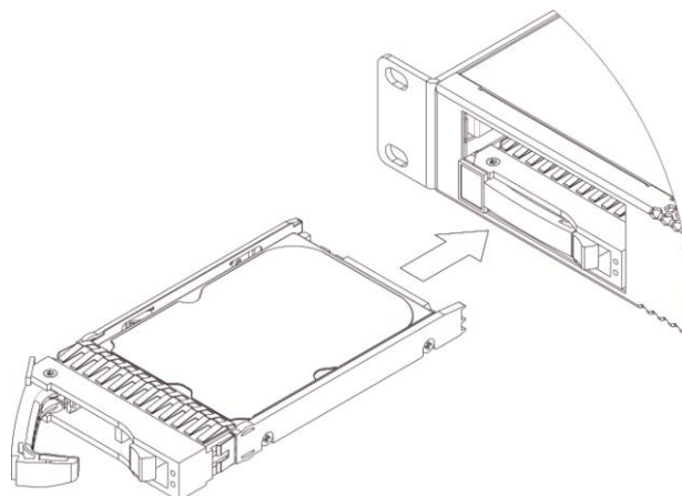
Рисунок 20 – Монтаж SATA-диска в корпус устройства
