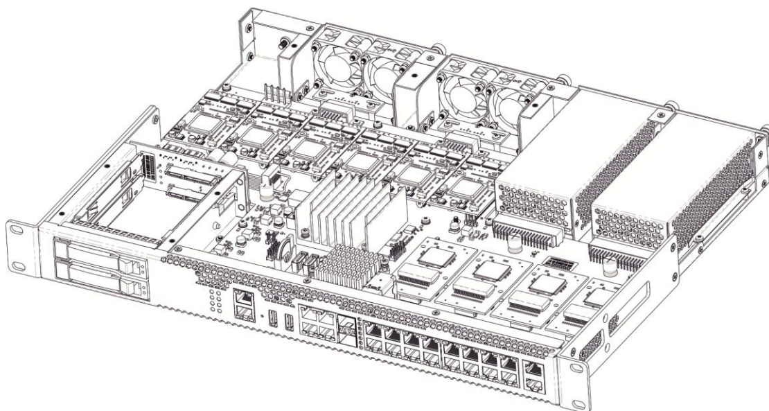
Рисунок 15 – Расположение submodule'ей в SMG-3016
