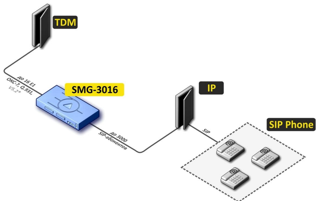
Рисунок 3 – Мини IP-PBX на базе SMG-3016
