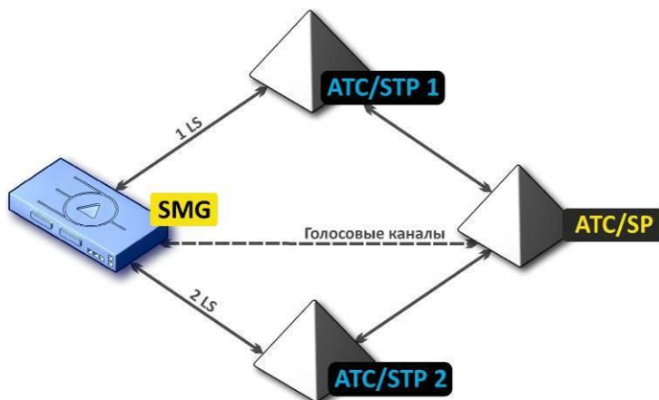
Рисунок 25 – Схема подключения SMG в комбинированном режиме
