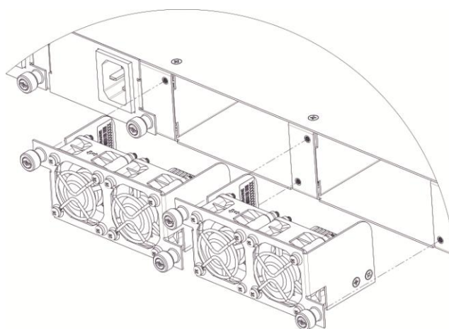
Рисунок 16 – Блок вентиляции SMG-3016. Крепление в корпус
