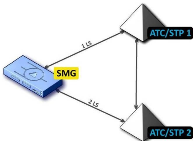
Рисунок 24 – Схема подключения SMG при работе в квазисвязанном режиме через АТС с STP
