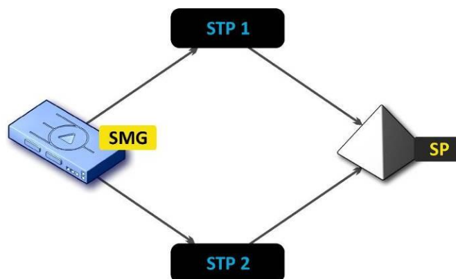
Рисунок 23 – Схема подключения SMG при работе в квазисвязанном режиме через STP
