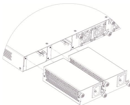
Рисунок 11 – Установка модулей питания
