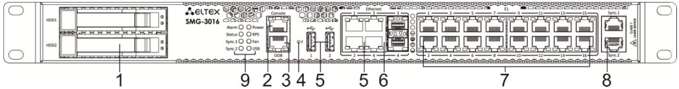
Рисунок 7 – Внешний вид передней панели SMG-3016
