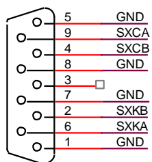
DB9
