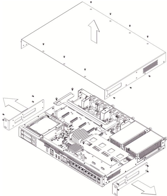
Рисунок 12 – Порядок вскрытия корпуса SMG-3016
