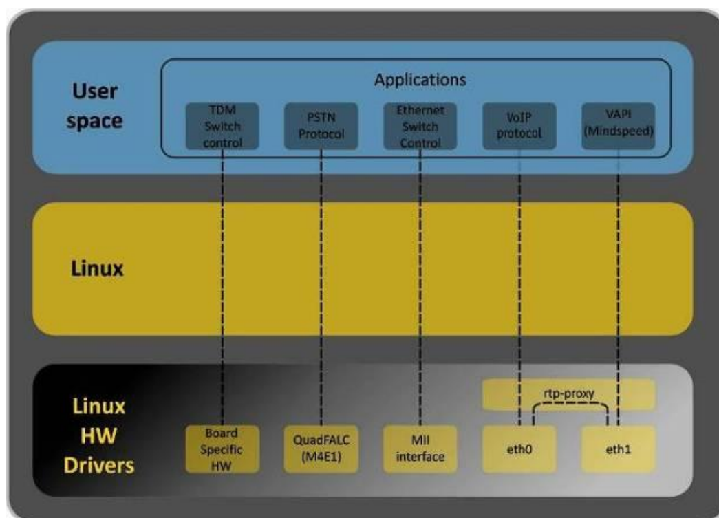
Рисунок 6 – Структура программного обеспечения SMG
