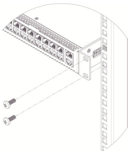
Рисунок 10 – Установка устройства в стойку
