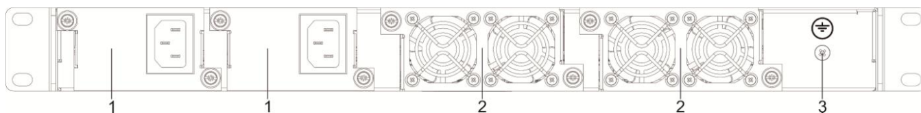
Рисунок 8 – Внешний вид задней панели SMG-3016
