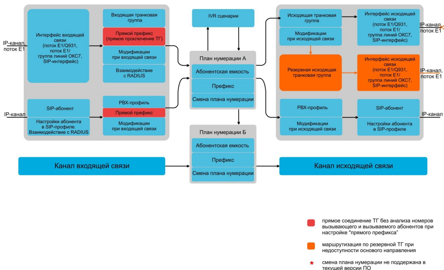
Рисунок 29 – Взаимосвязь параметров маршрутизации, абонентов и СЛ
