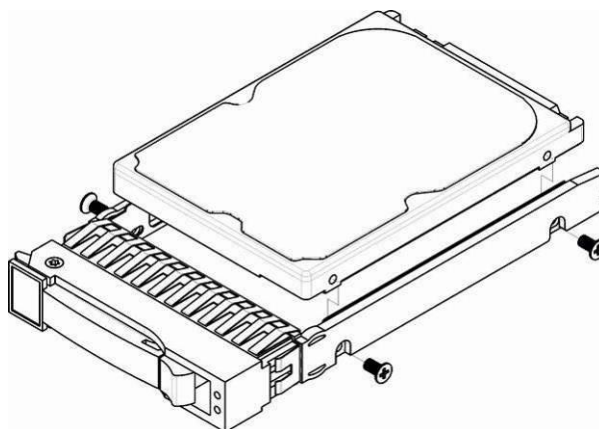
Рисунок 19 – Крепление SATA-диска в лоток направляющих салазок
