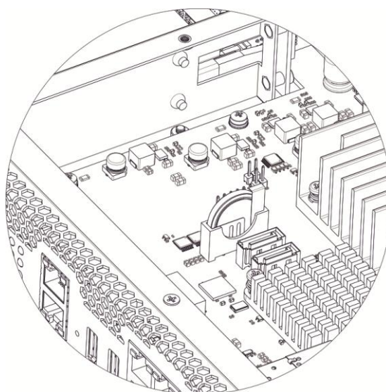
Рисунок 21 – Положение батарейки RTC для SMG-3016
