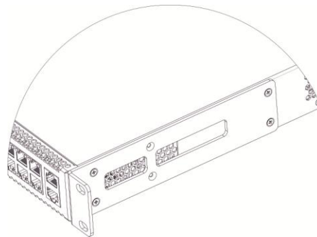
Рисунок 9 – Крепление кронштейнов
