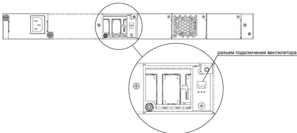
Рисунок 17 – Разъем для подключения вентилятора
