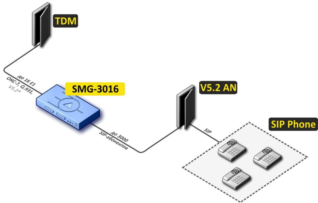
Рисунок 4 – Вынос V5.2 AN на базе SMG-3016
