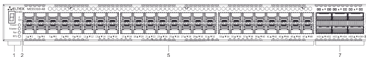
Рисунок 27 – Передняя панель MES5310-48
