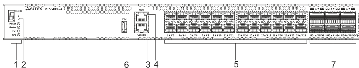
Рисунок 28 – Передняя панель MES5400-24
