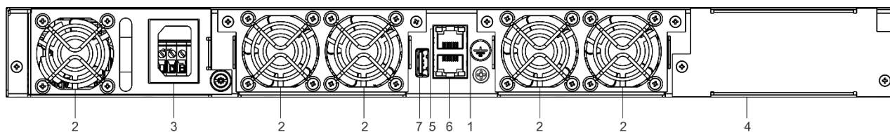
Рисунок 52 – Задняя панель MES5300-48, MES5305-48, MES5310-48
