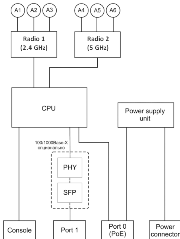
Рисунок 2 – Структурная схема WOP-12ac
