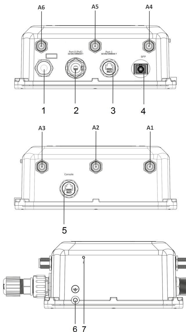
Рисунок 1 – Внешний вид боковых панелей WOP-12ас
