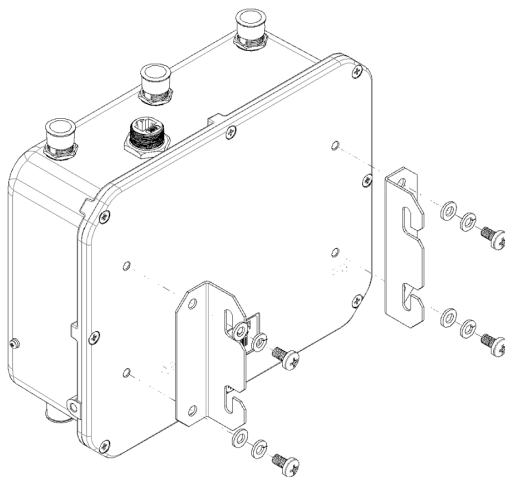
Рисунок 7 – Крепление кронштейнов к устройству
