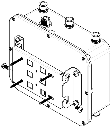
Рисунок 13 – Крепление устройства на стене
