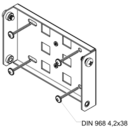
Рисунок 11 – Крепление кронштейна на стене
