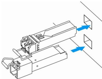
Рисунок 3.5 – Установка SFP-трансиверов
