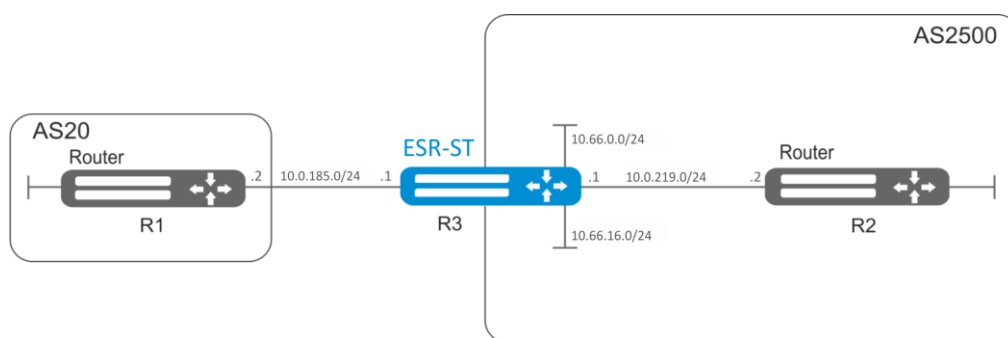
Рисунок 9.16 – Схема сети
