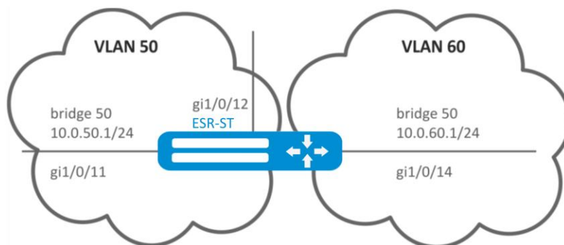
Рисунок 9.11 – Схема сети
