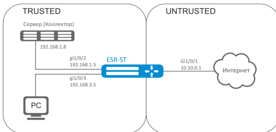
Рисунок 9.26 – Схема сети
