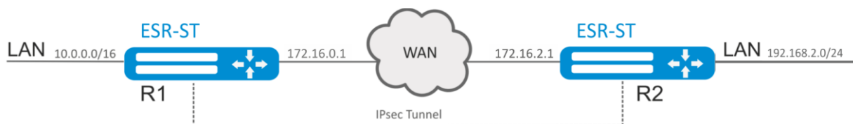
Рисунок 8.1 – Схема сети
