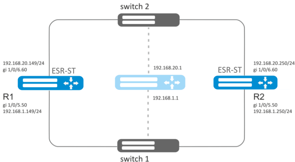
Рисунок 9.29 – Схема сети
