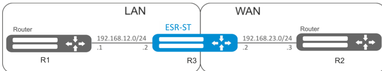
Рисунок 9.7 – Схема сети
