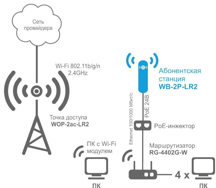
Функциональная схема использования WB-2P-LR2 с маршрутизатором
