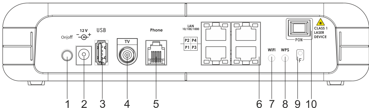
Рисунок 6 – Внешний вид задней панели NTU-RG-5421G-Wac
