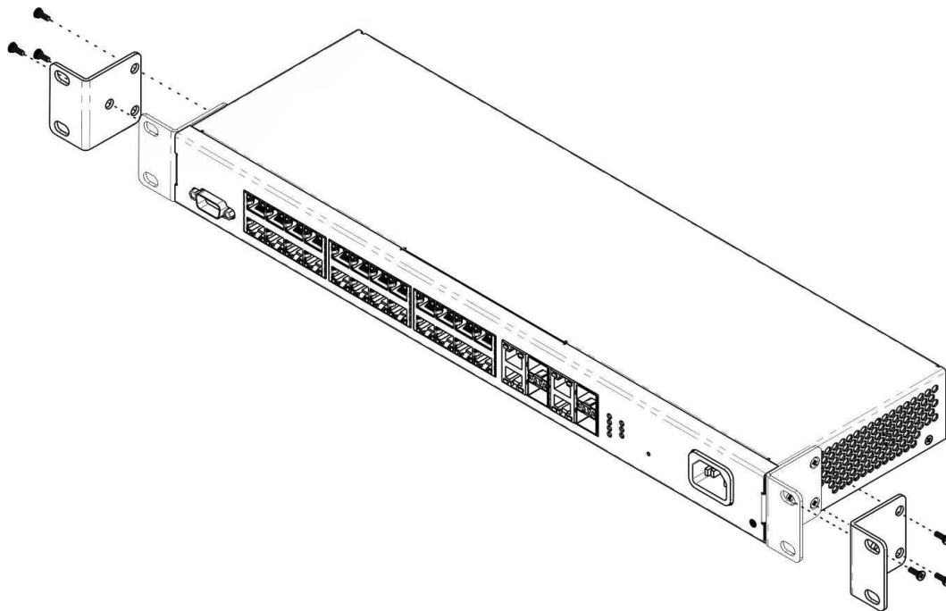
Рисунок 21 – Крепление кронштейнов
