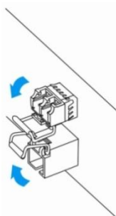
Рисунок 27 – Открытие защелки SFP-трансиверов
