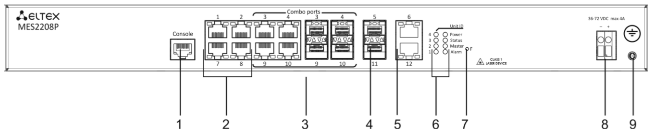
Рисунок 12 – MES2208P, передняя панель
