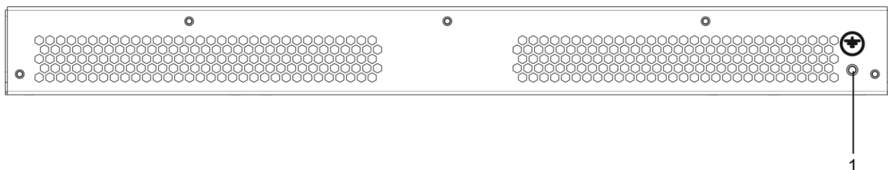
Рисунок 11 – MES1124M, MES2124M, задняя панель
