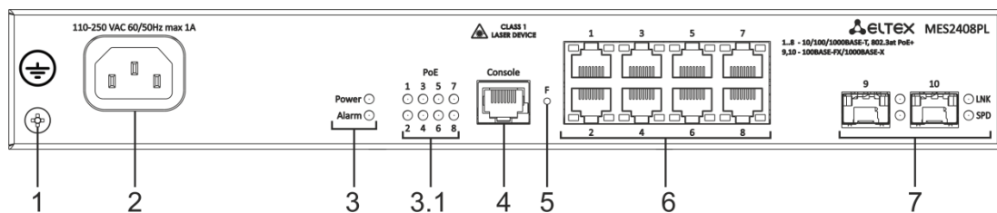
Рисунок 10 – Передняя панель MES2408PL
