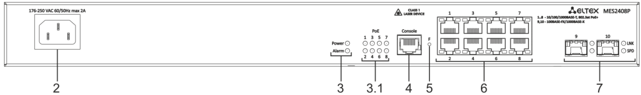
Рисунок 8 – Передняя панель MES2408P AC
