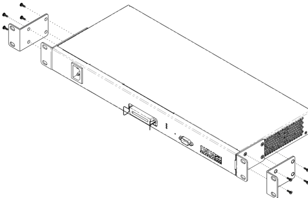
Рисунок 7 – Крепление кронштейнов
