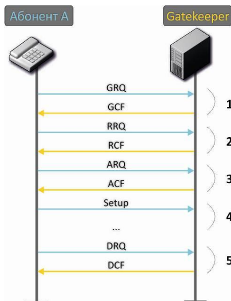
Рисунок 19 – Алгоритм вызова через гейткипер
