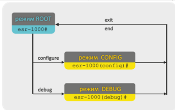
Рисунок 1 – Верхний уровень иерархии режимов команд
