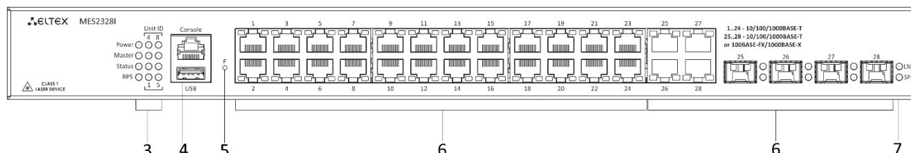
Рисунок 15 — Передняя панель MES2328I
