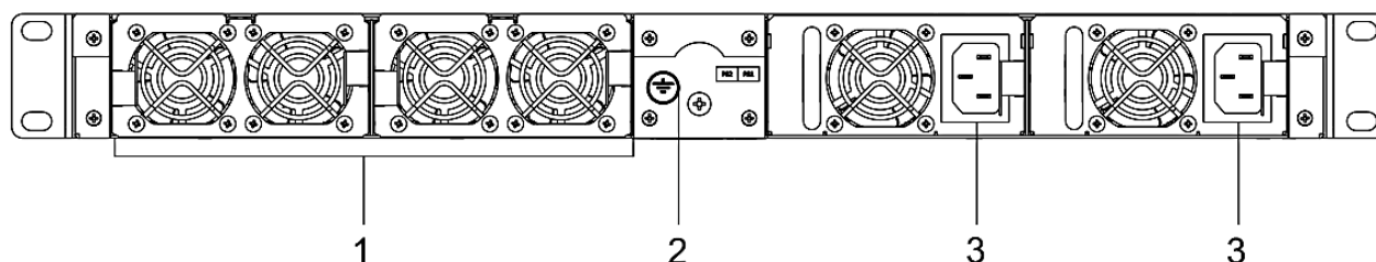
Рисунок 35 — Задняя панель MES2348P
