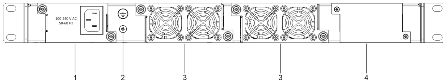
Рисунок 14 – Задняя панель ESR-3200L
