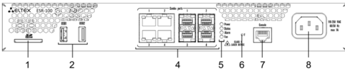
Рисунок 41 – Передняя панель ESR-100
