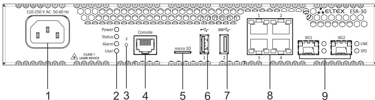
Рисунок 53 – Передняя панель ESR-30
