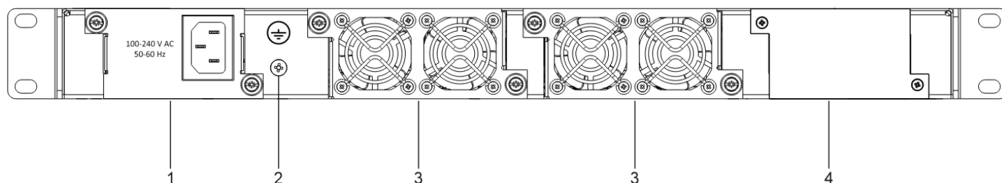
Рисунок 18 – Задняя панель ESR-3200
