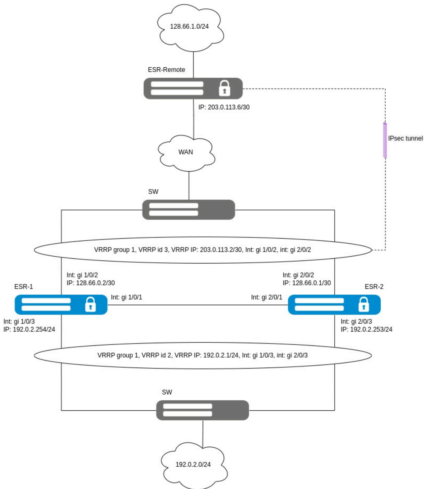
Схема реализации Policy-based IPsec VPN
