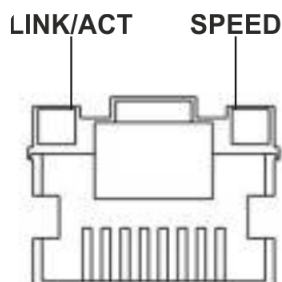
Рисунок 95 – Расположение индикаторов разъема RJ-45
