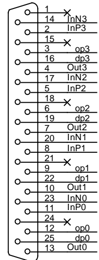
Модуль 4ТЛГ
