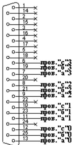
Модуль 4СЛУ
