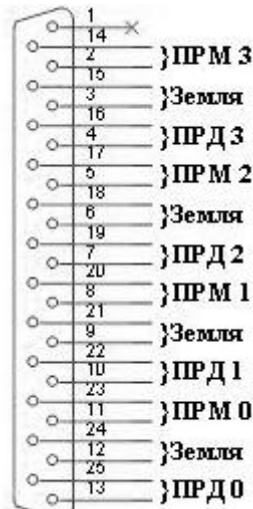
Субмодуль М4Е1
