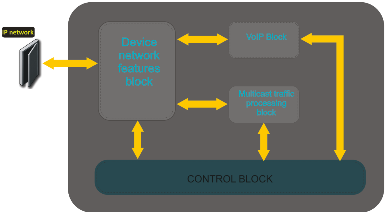
Fig. 3 – TAU-8.IP function diagram
