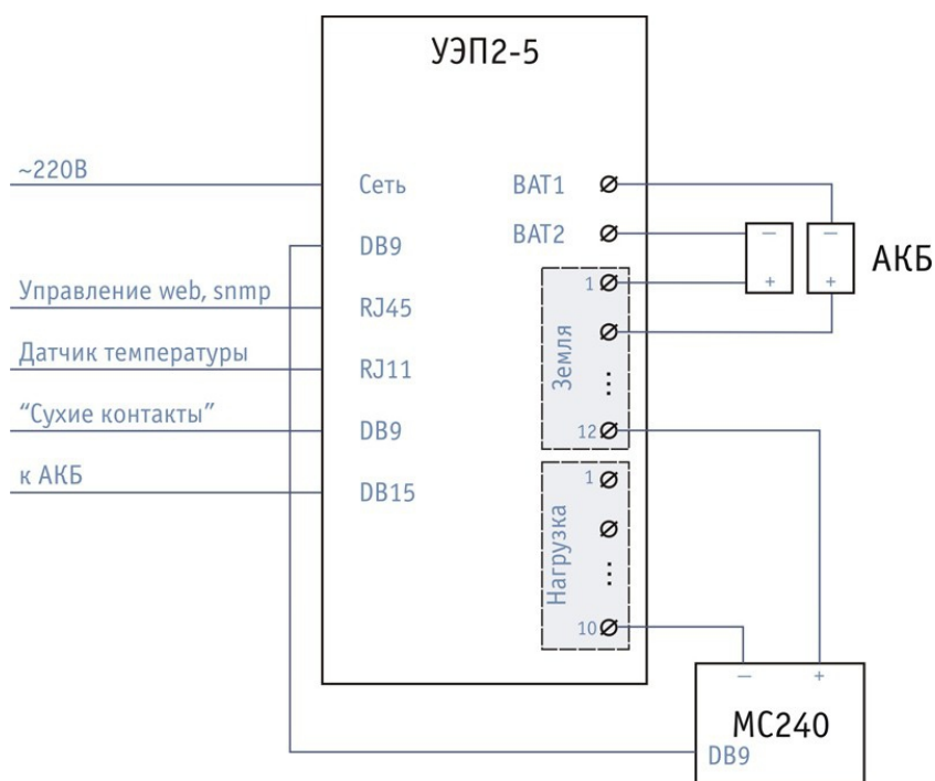
Рисунок 3 – Схема включения УЭП2-5
