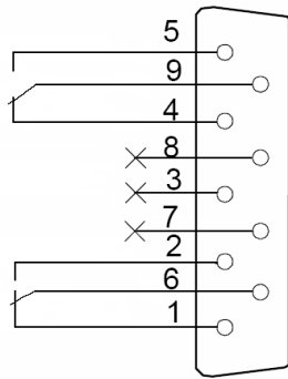
разъем Alarm
