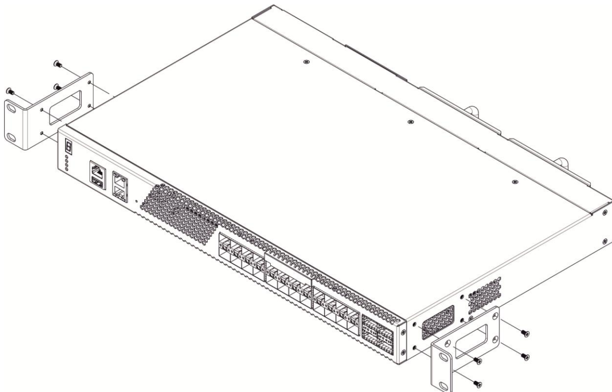
Рисунок 32 – Крепление кронштейнов
