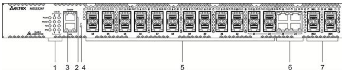
Рисунок 2 – Передняя панель MES3324F
