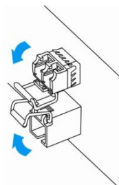
Рисунок 39 – Открытие защелки SFP-трансиверов
