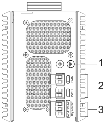
Рисунок 26 – Верхняя панель MES3508P
