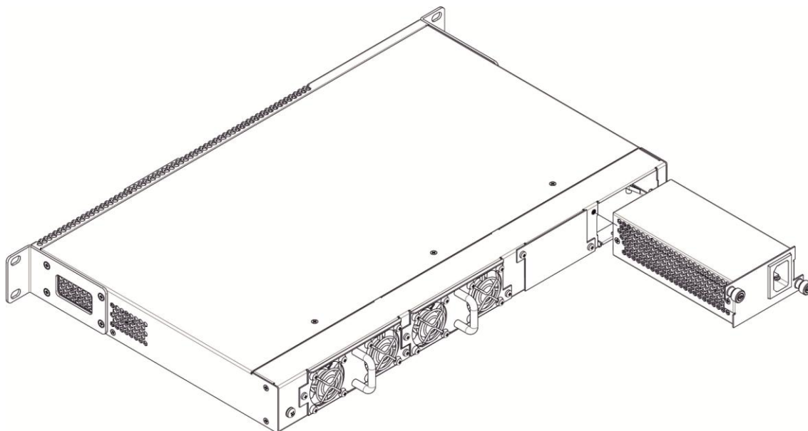
Рисунок 35 – Установка модулей питания.
