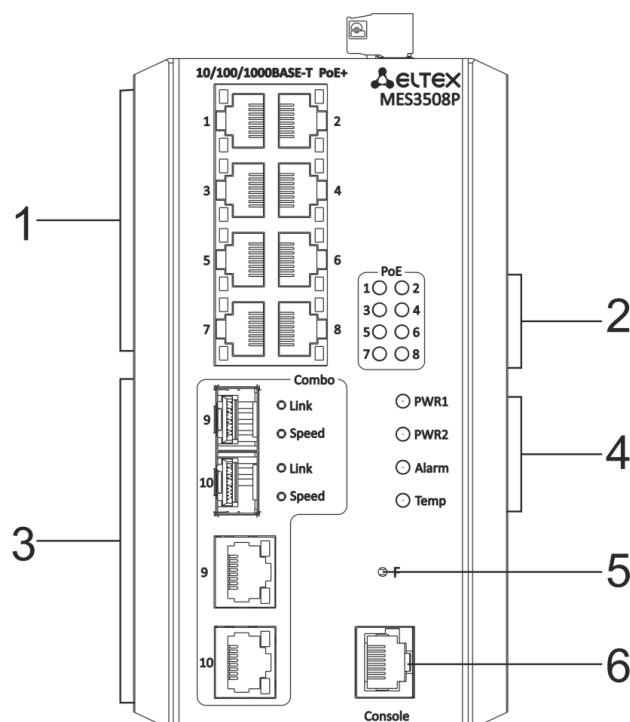
Рисунок 19 – Передняя панель MES3508P
