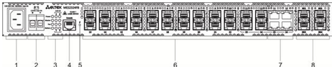
Рисунок 10 – MES2324FB, передняя панель
