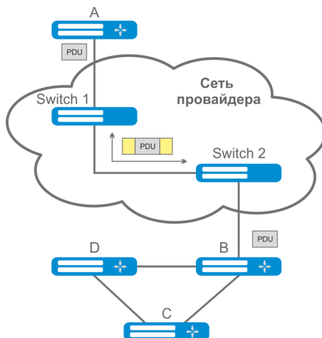
Рисунок 42 – Пример работы функции L2PT
