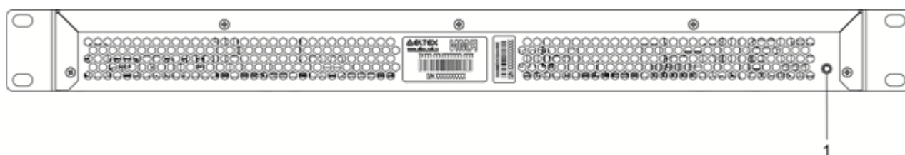
Рисунок 22 – Задняя панель MES2324, MES2324B, MES2324F DC, MES2324P
