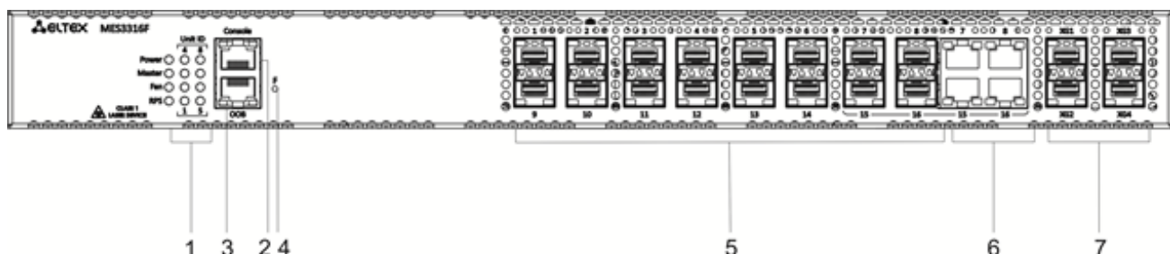
Рисунок 4 – Передняя панель MES3316F
