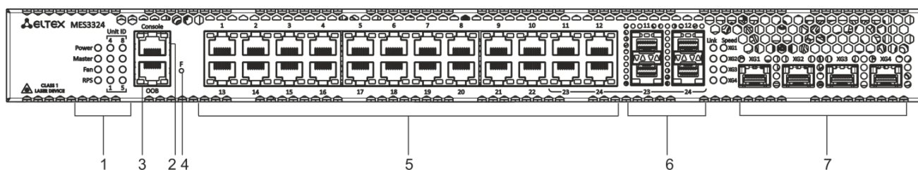
Рисунок 3 – Передняя панель MES3324
