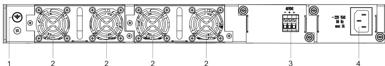
Рисунок 20 – Задняя панель MES5324
