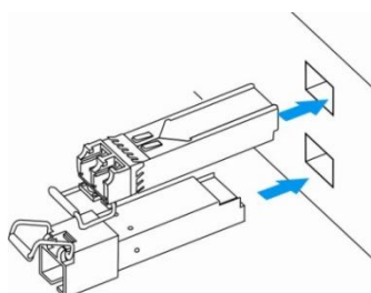
Рисунок 37 – Установка SFP-трансиверов
