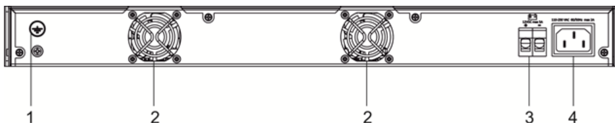
Рисунок 24 – Задняя панель MES2348B
