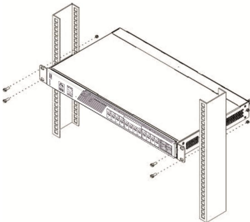
Рисунок 33 – Установка устройства в стойку
