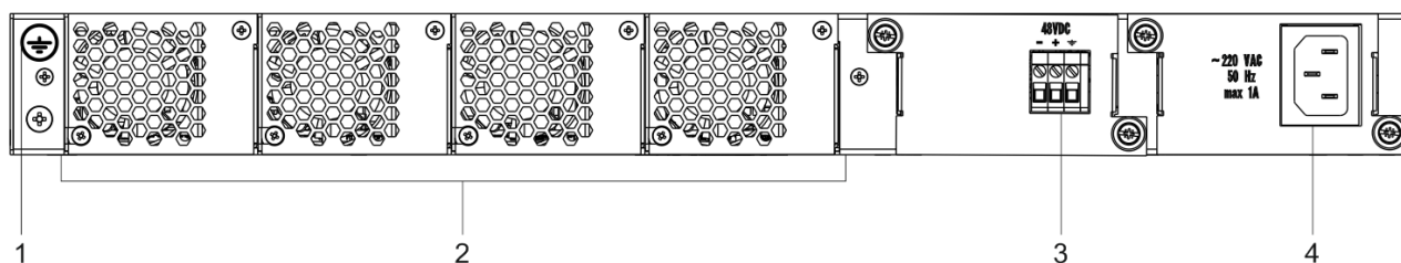
Рисунок 21 – Задняя панель MES3324F, MES3348, MES3348F, MES3324, MES3308F, MES3316F
