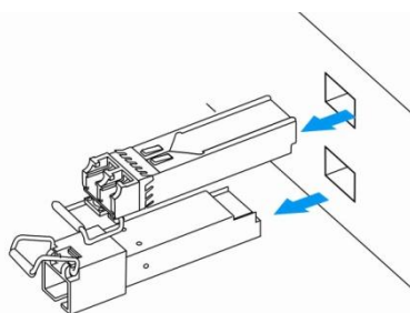
Рисунок 40 – Извлечение SFP-трансиверов
