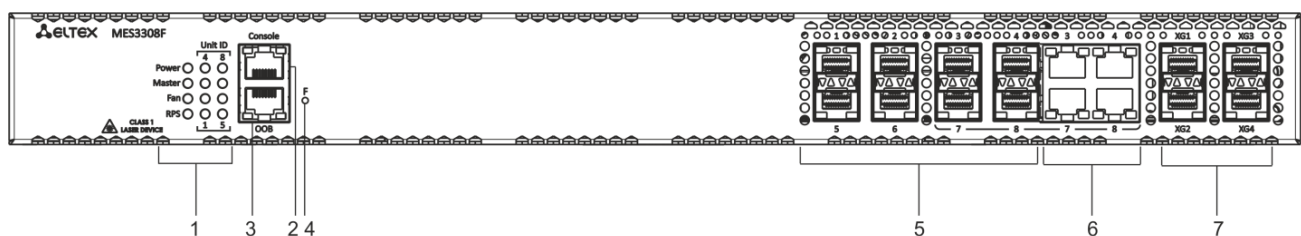
Рисунок 5 – Передняя панель MES3308F
