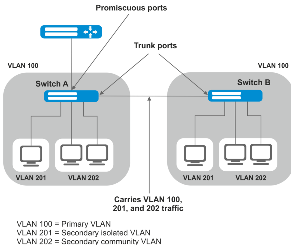
Рисунок 41 – Пример работы технологии Private VLAN
