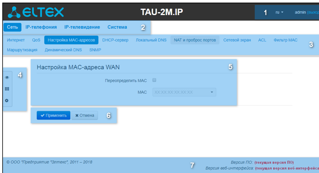
Рисунок 7 – Элементы навигации Web-конфигуратора
