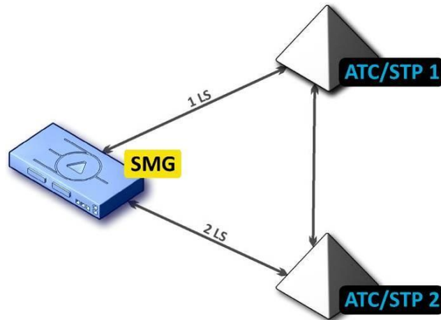
Рисунок 36 – Схема подключения SMG при работе в квазисвязанном режиме через АТС с STP LS – группа линий ОКС-7 (Link Set)
