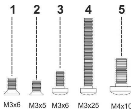
Рисунок 19 – Типы болтов для сборки SMG
