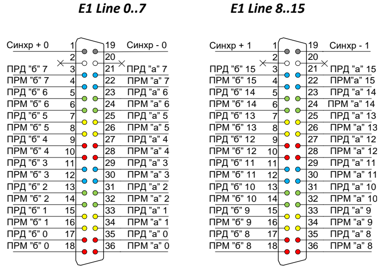
Рисунок 39 – Назначение контактов разъемов E1 Line
