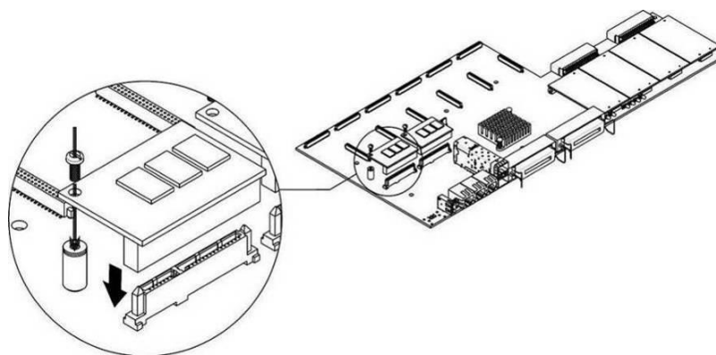
Рисунок 28 – Монтаж SSD-накопителя
