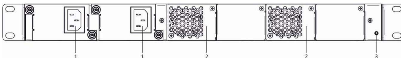
Рисунок 11 – Внешний вид задней панели SMG-1016M
