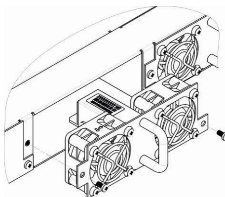
Рисунок 23 – Блок вентиляции SMG-1016M. Крепление в корпус
