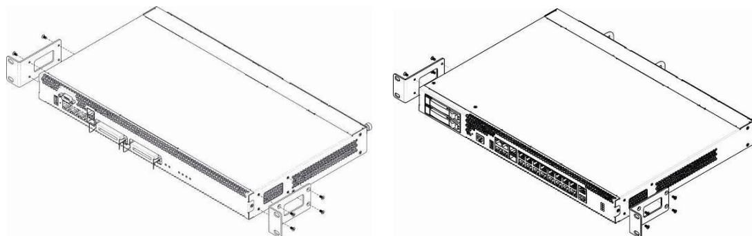
Рисунок 14 – Крепление кронштейнов для SMG-1016M (слева) и SMG-2016 (справа)
