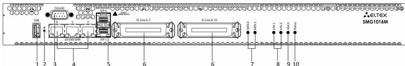
Рисунок 10 – Внешний вид передней панели SMG-1016M
