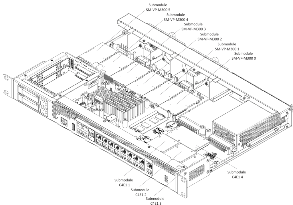
Рисунок 22 – Расположение submodule в SMG-2016
