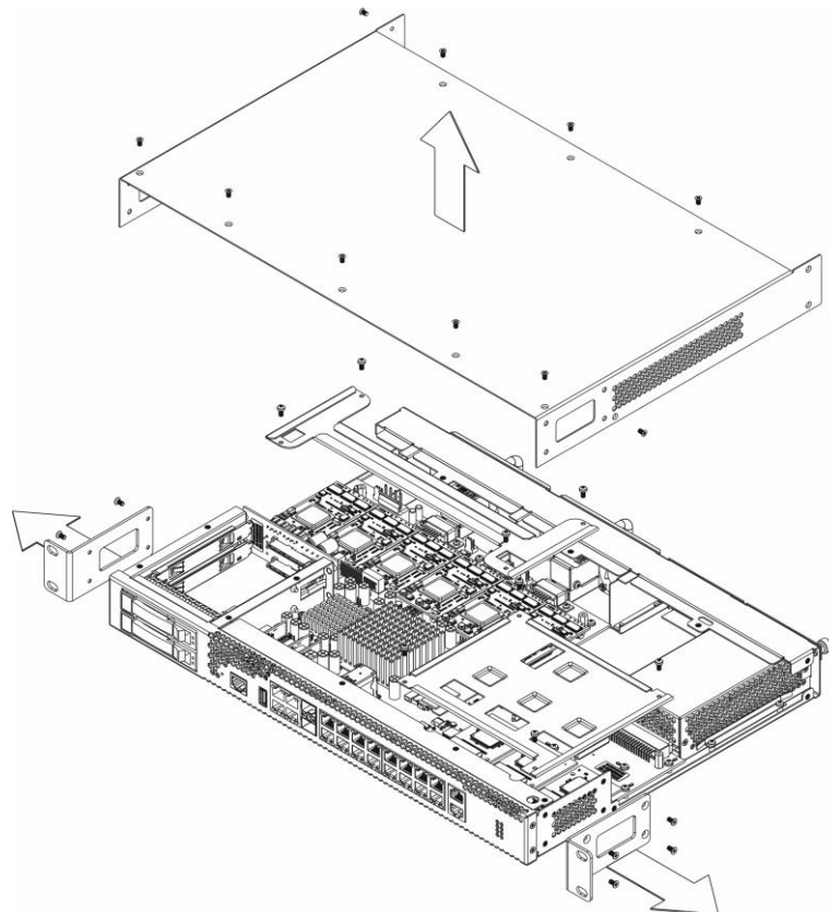
Рисунок 18 – Порядок вскрытия корпуса SMG-2016
