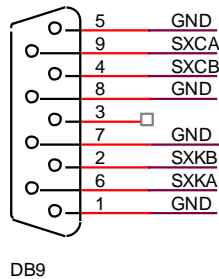
Рисунок 40 – Назначение контактов разъема Console
