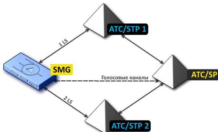
Рисунок 37 – Схема подключения SMG в комбинированном режиме
