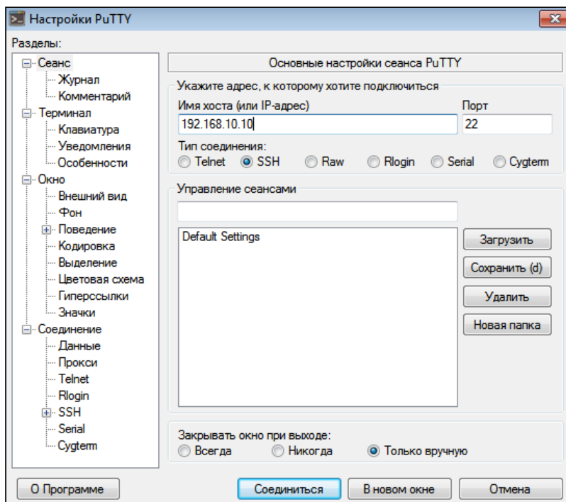
Рисунок 2 – Запуск SSH-клиента
